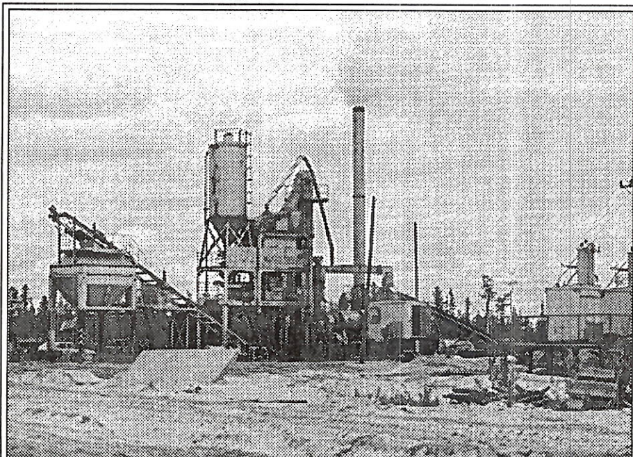
Асфальтовый завод
