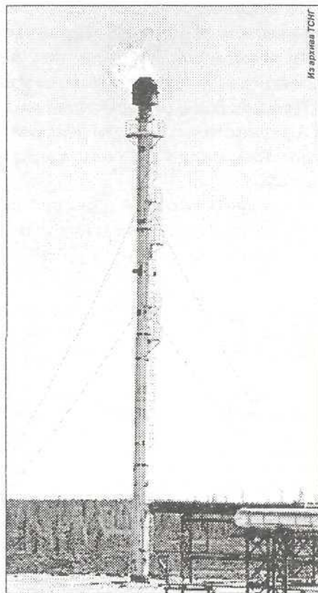
Факельное хозяйство
